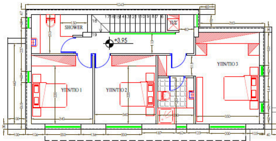
Κατοψη οροφου
